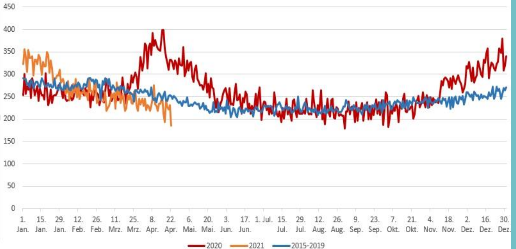
Schweden: Todesfallzahlen pro Tag 2020/2021 vs. 2015-2019
